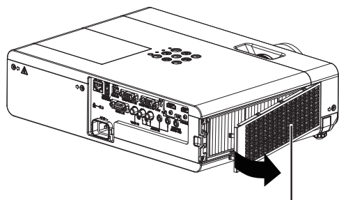
Рис. 1 Крышка воздушного фильтра
