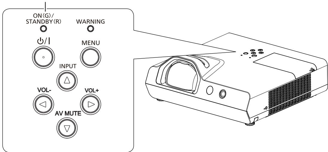
Индикатор питания <ON(G)/STANDBY(R)>
